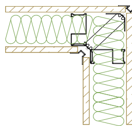
Eckausbildung in Holz
