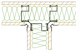
Wand- Wandanschluss in Holz
