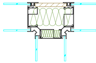
Wand- Wandanschluss in Glas
