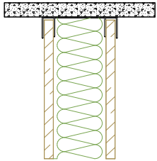
Decken- und Wandanschluss
