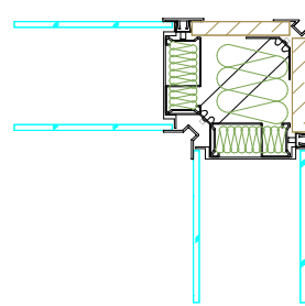
Wand- Wandanschluss in Glas
